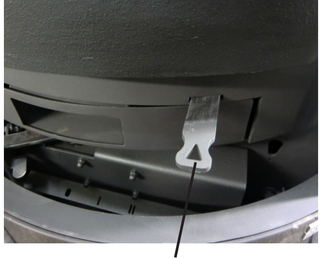
Regelhendel voor het vuurrooster
